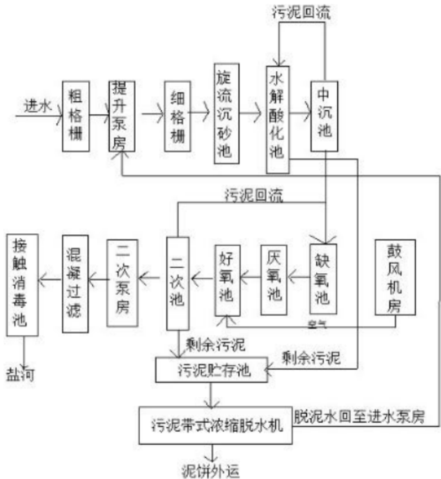
图 4-1 新渡片区污水处理厂污水处理工艺流程图
