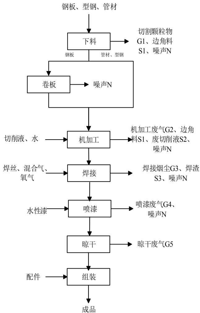
图 2-1 建设项目工艺流程图及产污示意图
